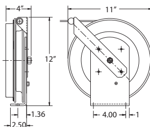
1472, 1473 Dimensions
