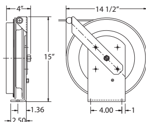
1471 Dimensions
